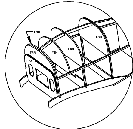
Step 4.2--cross brace
